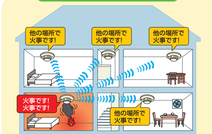
連動型住宅用火災警報器イメージ
